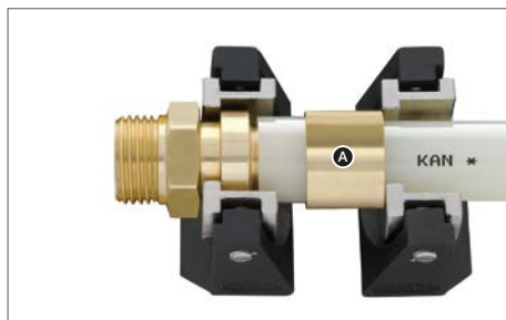
Montaż złączek z GZ i GW \text{Ø}12 \times 2 , \text{Ø}14 \times 2 , \text{Ø}18 \times 2 , \text{Ø}18 \times 2,5
