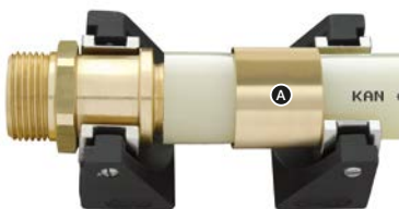
Монтаж соединителей с наружной и внутренней резьбой Ø25×3,5
