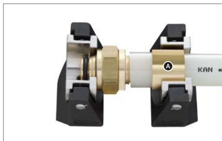
Montaż śrubunka z pierścieniem nasuwanym
