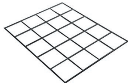
Mata z drutu 3 mm o wymiarach 1,2 m×2,1 m i rozstawie oczek 150×150 mm
