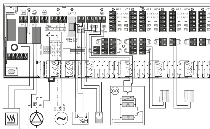
Rys. 71. Konfiguracja listwy elektrycznej Basic+ 230 V lub 24 V z modułem pompowym, modułem kotła i urządzeniami peryferiów.
