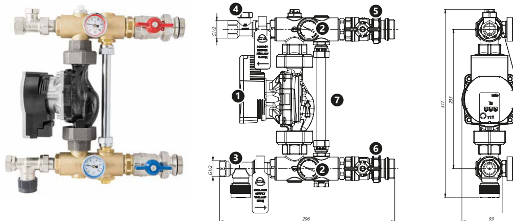
Rys. 53. Budowa zespołu pompowego KAN-therm.
