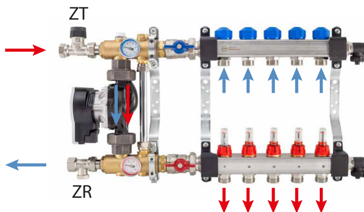
Rys. 56. Rozdzielacz z układem mieszającym USFP – kierunki przepływów.
