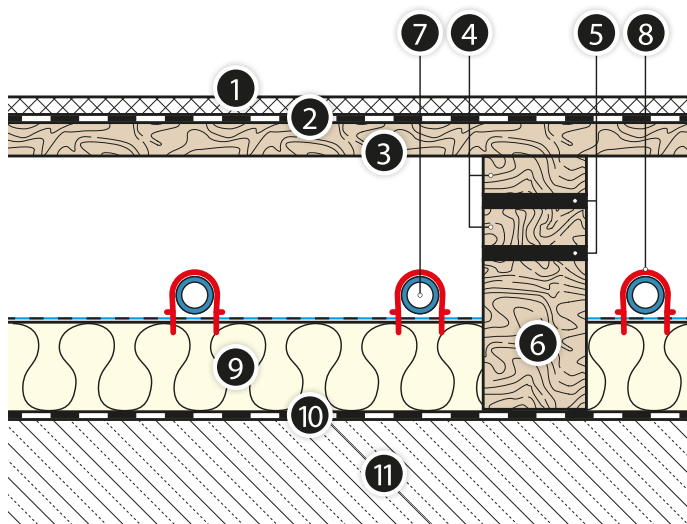
Rys. 32. Przekrój podłogi sportowej elastycznej powierzchniowo, z instalacją ogrzewania podłogowego wykonanego z elementów systemu KAN-therm Tacker.
