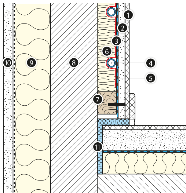
Rys. 36. Budowa instalacji ogrzewania ściennego KAN-therm TBS.
