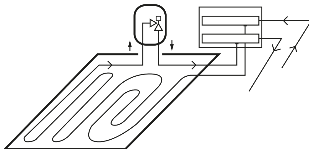
Rys. 76. Schemat działania – zespół umieszczony na powrocie.
