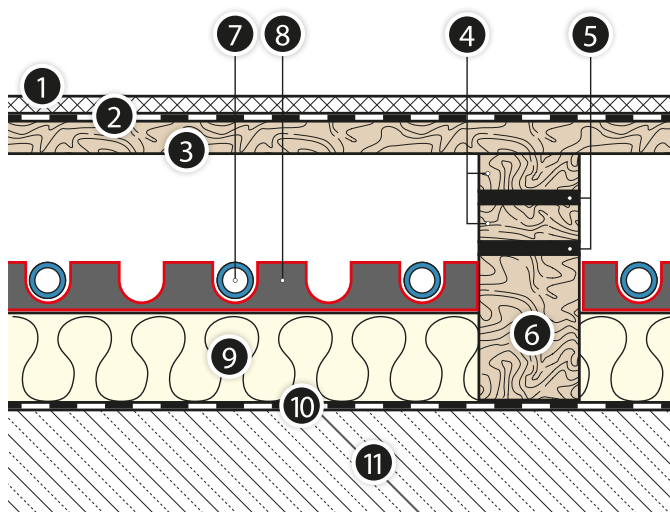
Rys. 33. Przekrój podłogi sportowej elastycznej powierzchniowo, z instalacją ogrzewania podłogowego wykonanego z elementów systemu KAN-therm Rail.
