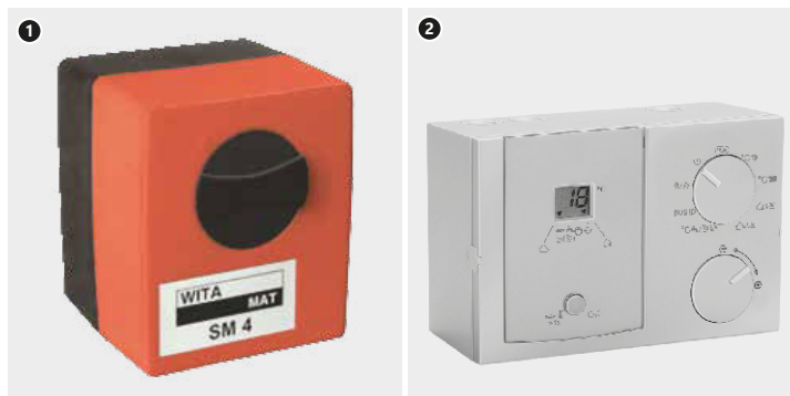
Rys. 51. Elementy sterujące centralnego układu z mieszaniem KAN-therm (siłownik SM4 (1) i regulator pogodowy (2)).
