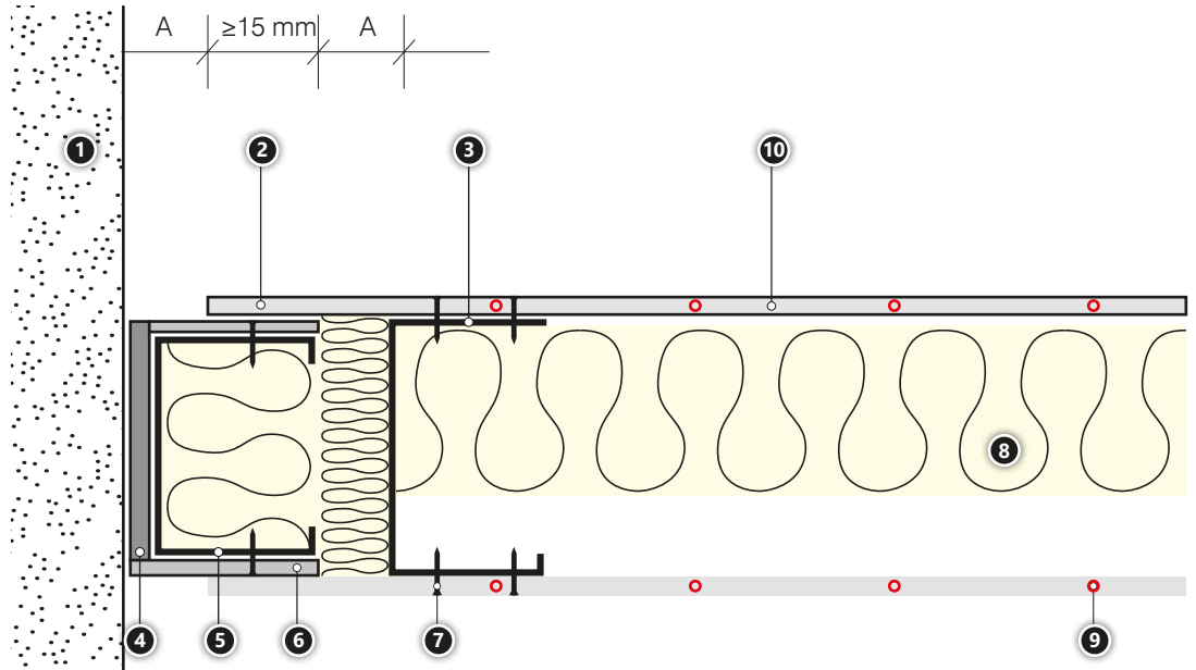
Rys. 41. Połączenie ślizgowe ze ścianą.
