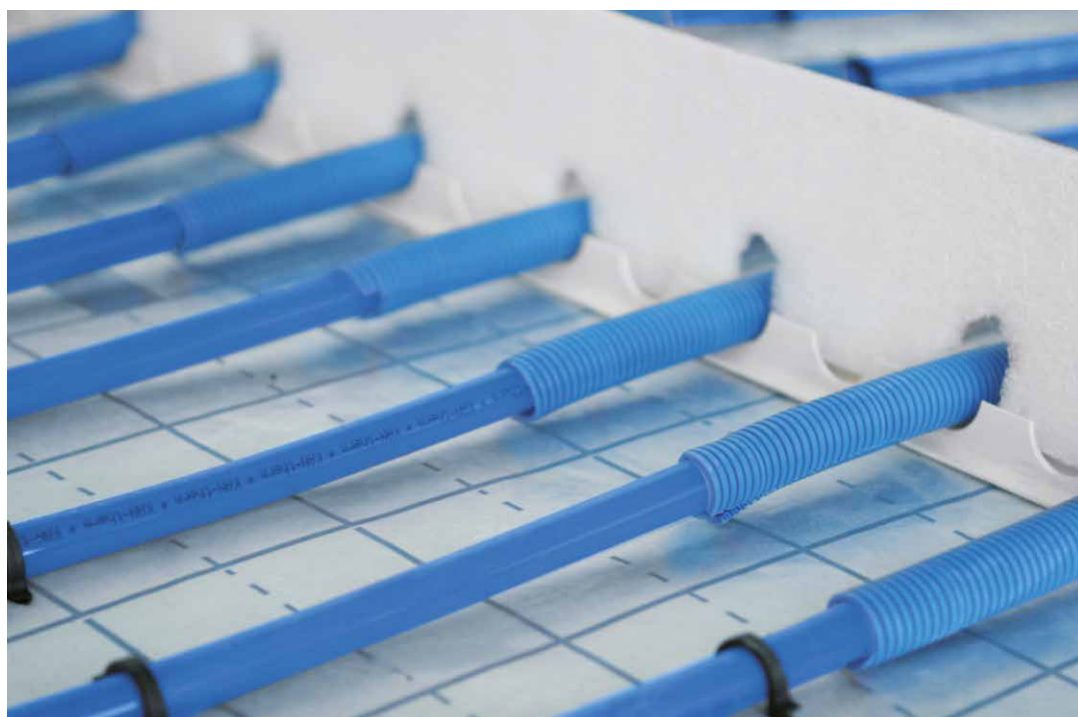
Rys. 17. Profil dylatacyjny - sposób prowadzenia rur tranzytowych przez dylatację.
