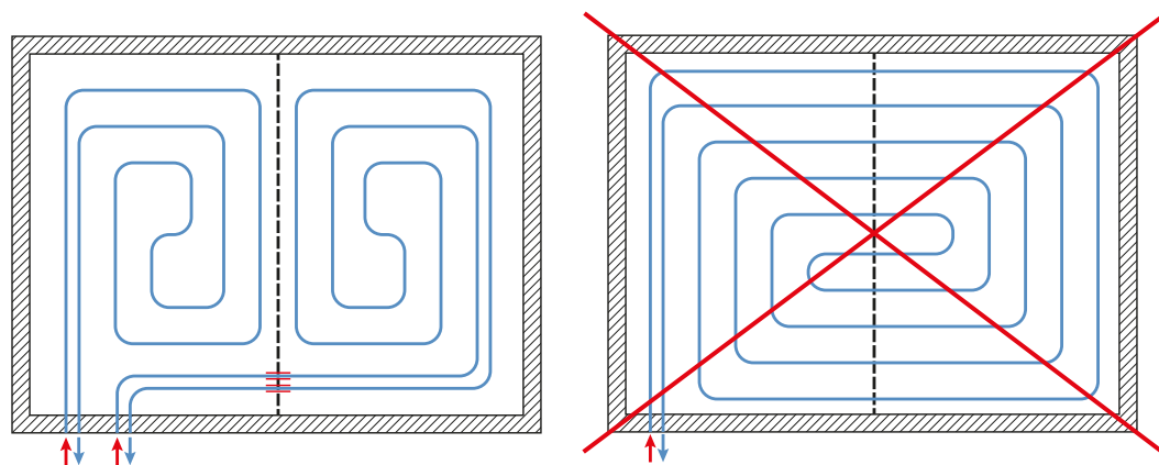
Rys. 19. Prawidłowy i nieprawidłowy podział pola grzewczego szczeliną dylatacyjną.
