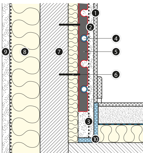
Rys. 35. Budowa instalacji ogrzewania/chłodzenia ściennego KAN-therm Rail.
