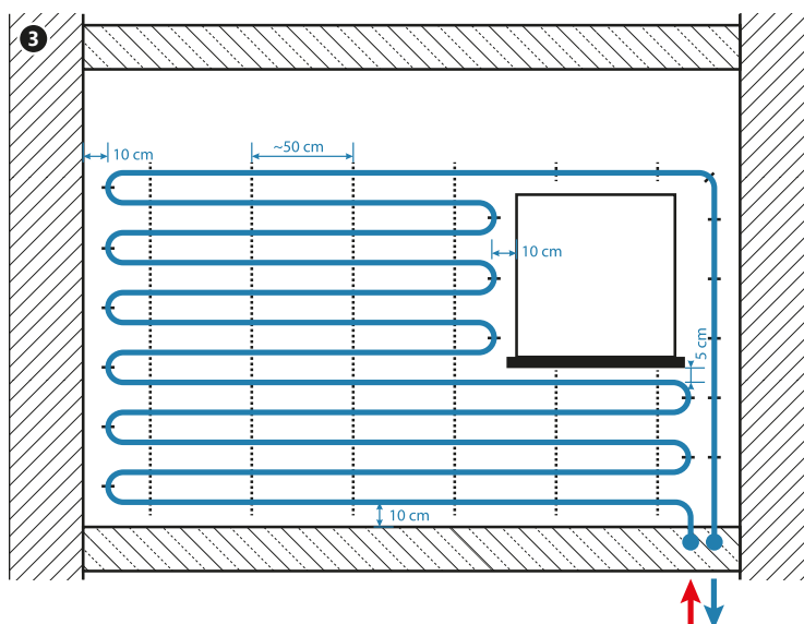
Rys. 34. Odległości montażowe w ogrzewaniu ściennym.
