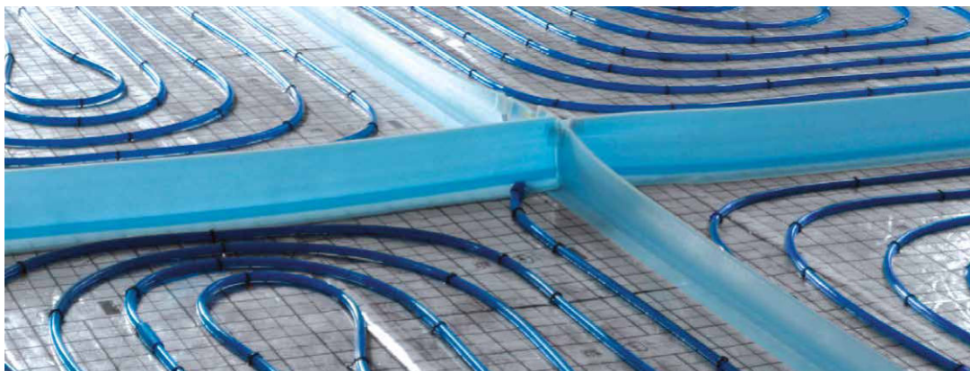
Rys. 14. Podział pól grzewczych szczelinami dylatacyjnymi.
