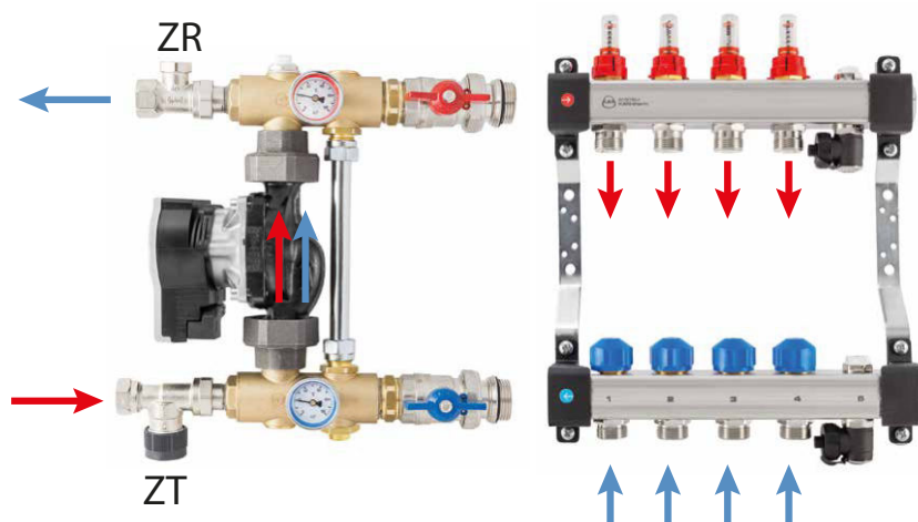
Rys. 57. Grupa pompowa stałowartościowa z rozdzielaczem UFST – kierunki przepływów.
