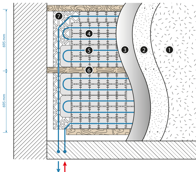
Rys. 37. Przekrój instalacji ogrzewania ściennego KAN-therm TBS.
