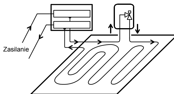
Rys. 6 Zestaw pomieszczeniowy – na zasilaniu
