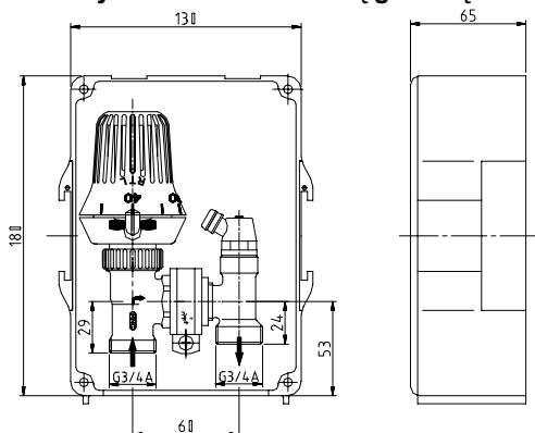
Rys. 1: RTL z widoczną głowicą
