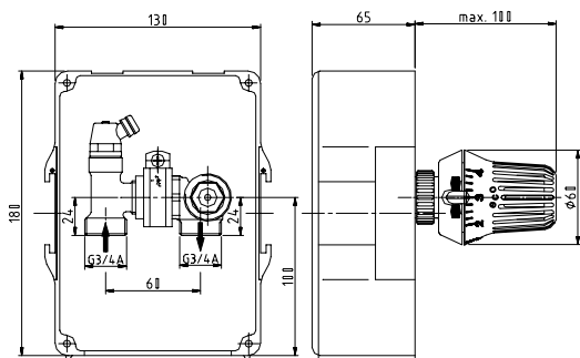
Rys. 3: Zestaw pomieszczeniowy
